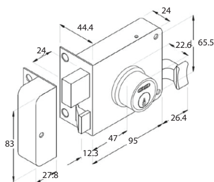
DIMENSIONES (mm)
