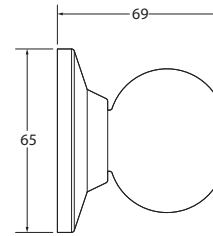
DIMENSIONES (mm)
