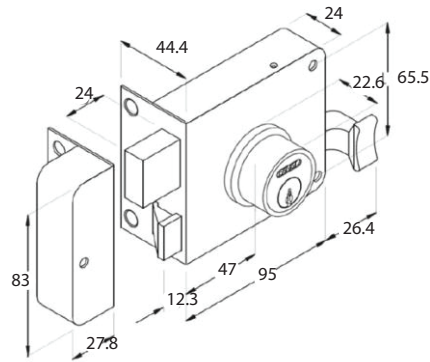
DIMENSIONES (mm)
