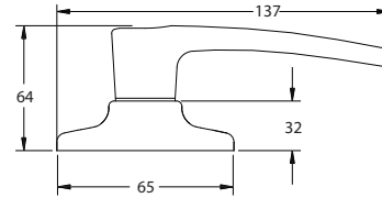
DIMENSIONES (mm)
